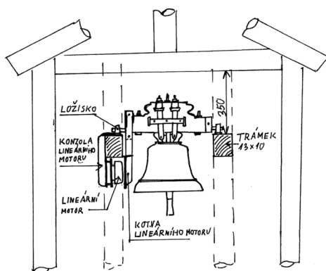
NÁRYS VEŽIČKA KAPLE INSTALACE ZVONU
